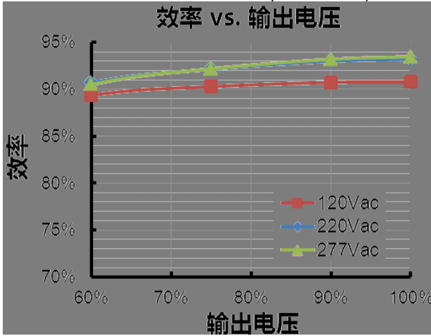
EUP-096S150ST (Io=1050mA)
