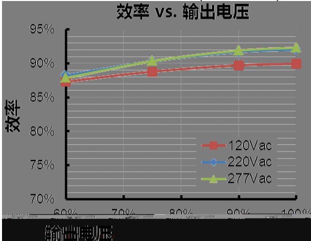
EUP-096S215ST( I_o=1750mA )
